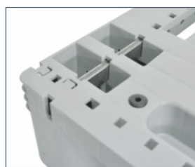
Stalowy profil wzmacniający na krótkim i długim boku
