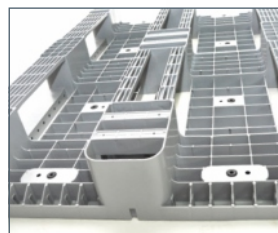
Możliwość zamontowania antypoślizgowych, gumowych korków na spodzie palety
