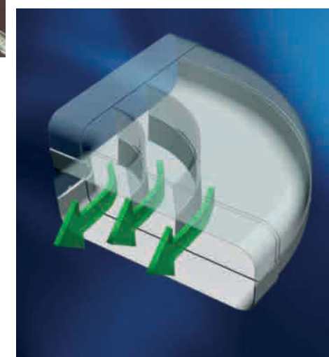
Die „Thermobox“ wird in den Mauerkästen integriert und bietet eine kontrollierte Wohnungslüftung (o.). Der „Compair flow“-Rohrbogen optimiert die Luftkanalsysteme, sodass deutlich weniger Druckverluste entstehen (u.).
