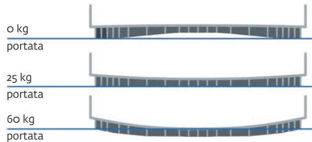
Fondo a cerchione 17 mm
