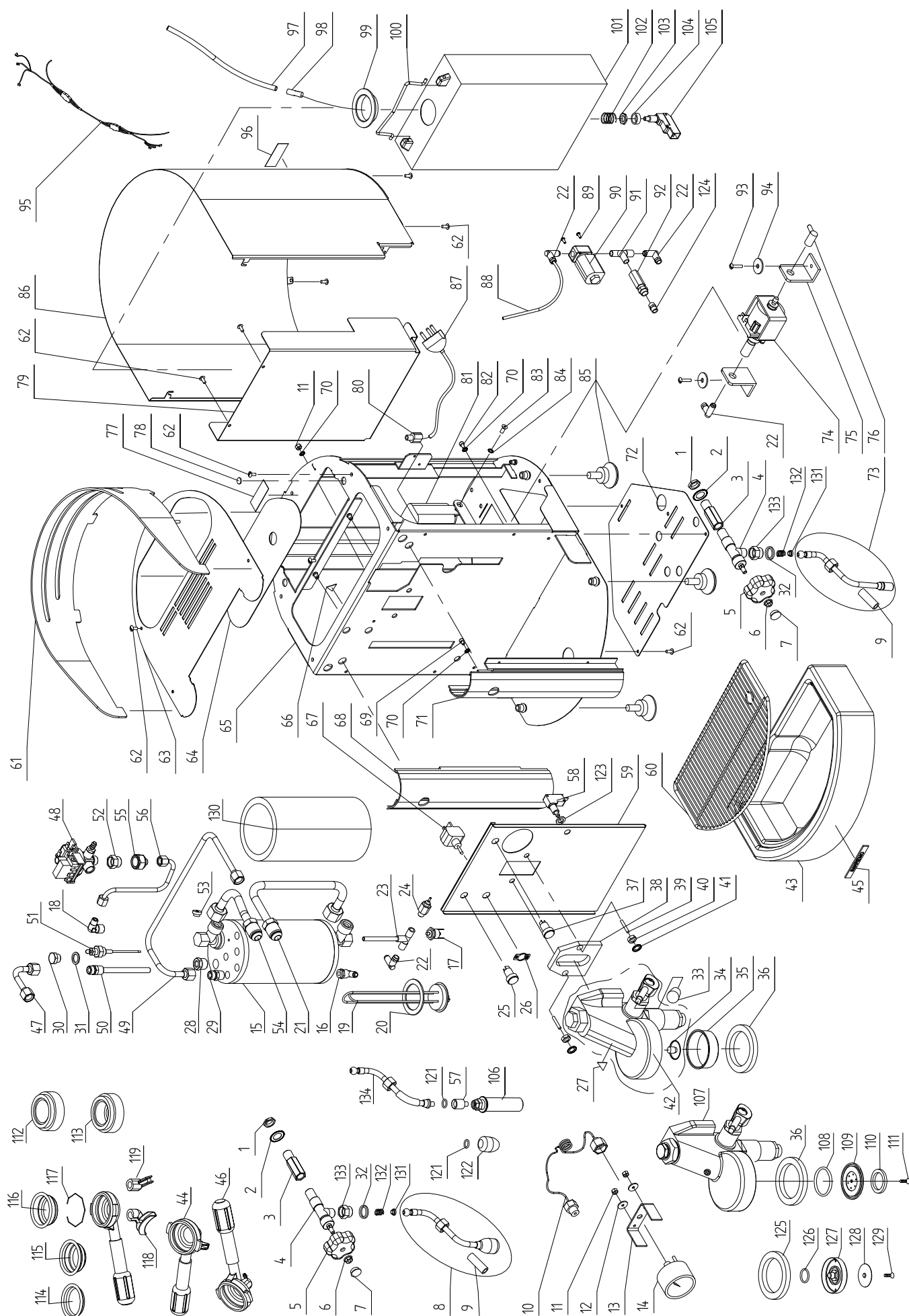
Schéma détaillé Mod. TREVISO - mise à jour.09/09
